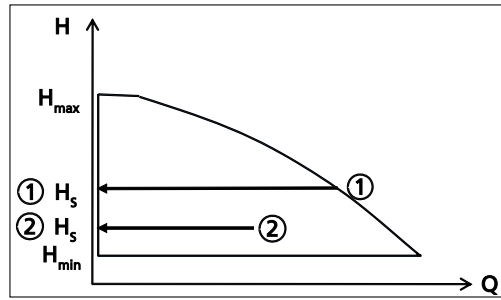
Abb. 13: Funktion Konstantdruckregelung
