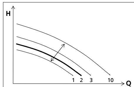
Abb. 19: Funktion Festdrehzahlbetrieb
