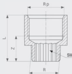
Reduzierstück - Rotguss oder Siliziumbronze Modell 3242
