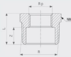
Reduzierstück - Rotguss oder Siliziumbronze Modell 3241
