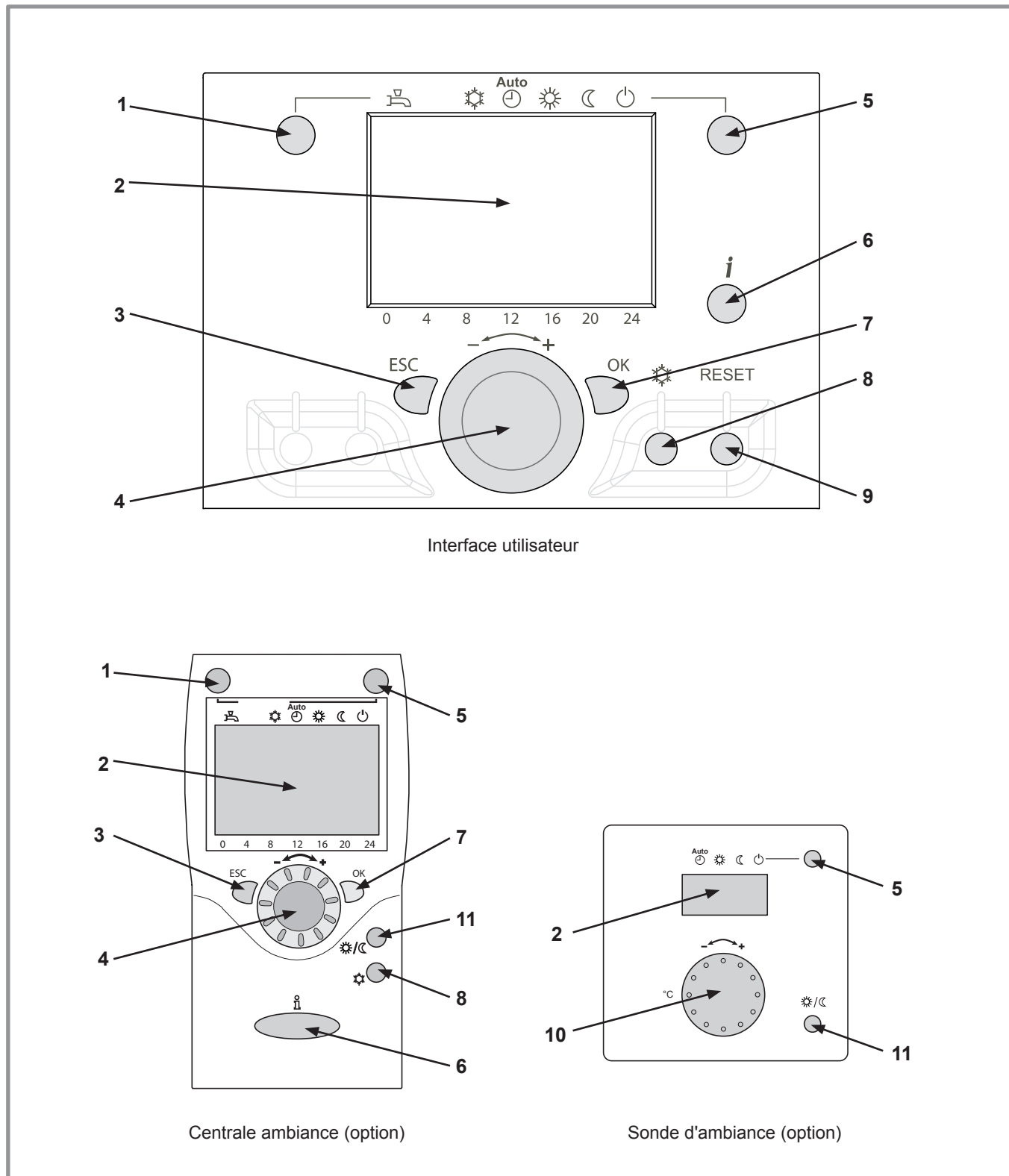
figure 2 - L'interface utilisateur, la centrale ambiance (option) et la sonde d'ambiance (option)
