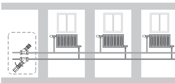
Kombi-3-Plus - Zonenregelung
