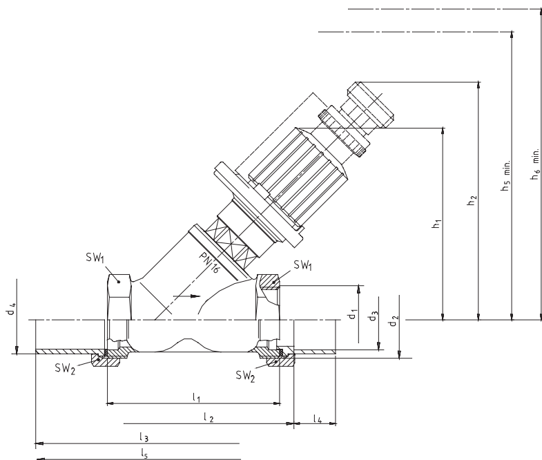
labelle 3. Baumaße V5010 Kombi-3-plus blau
