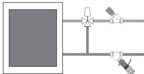
Kombi-3-Plus - Lufterhitzer
